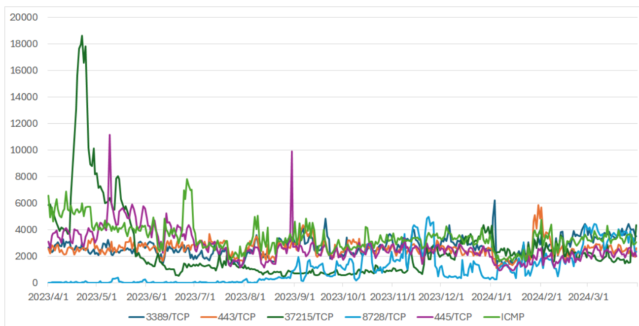
[図 1-5 : TSUBAME で観測された宛先ポートの上位 6 位から 10 位の packets 数 (2023 年 4 月 1 日～2024 年 3 月 31 日)]
