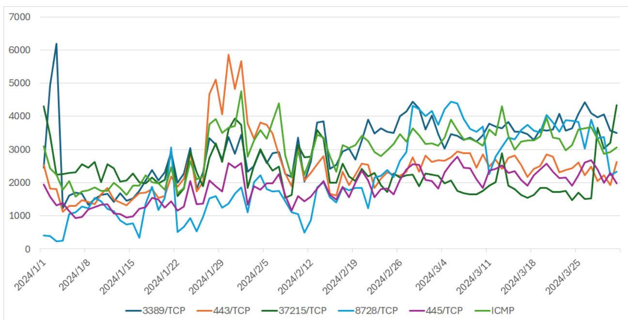
〔図 1-3：TSUBAME で観測された宛先ポートの上位 6 位から 10 位のパケット数（2024 年 1 月 1 日～3 月 31 日）〕
