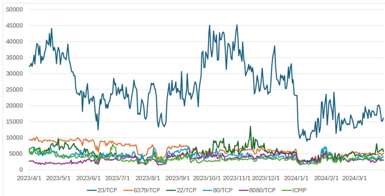
[図 1-4 : TSUBAME で観測された宛先ポートの上位 1 位から 5 位の packets 数 (2023 年 4 月 1 日～2024 年 3 月 31 日)]
