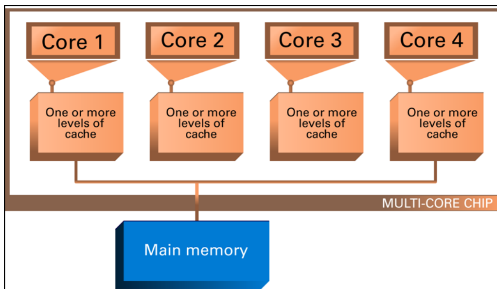
図 2: 現代の共有メモリ型マルチプロセッサのアーキテクチャ
