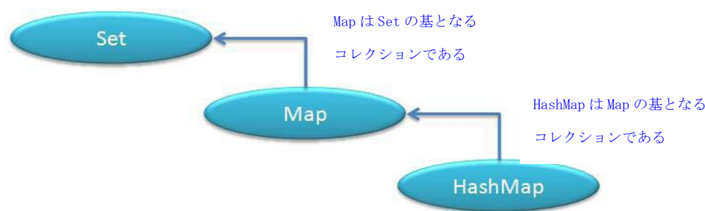
図 4: 違反コード例におけるコレクションビューと基となるコレクションの関係
