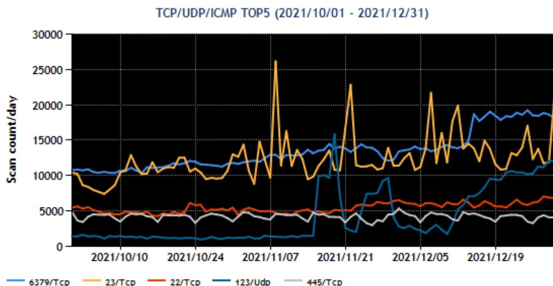
[図 1 : 2021 年 10～12 月のポート番号宛のパケット観測数トップ 5 の推移]
