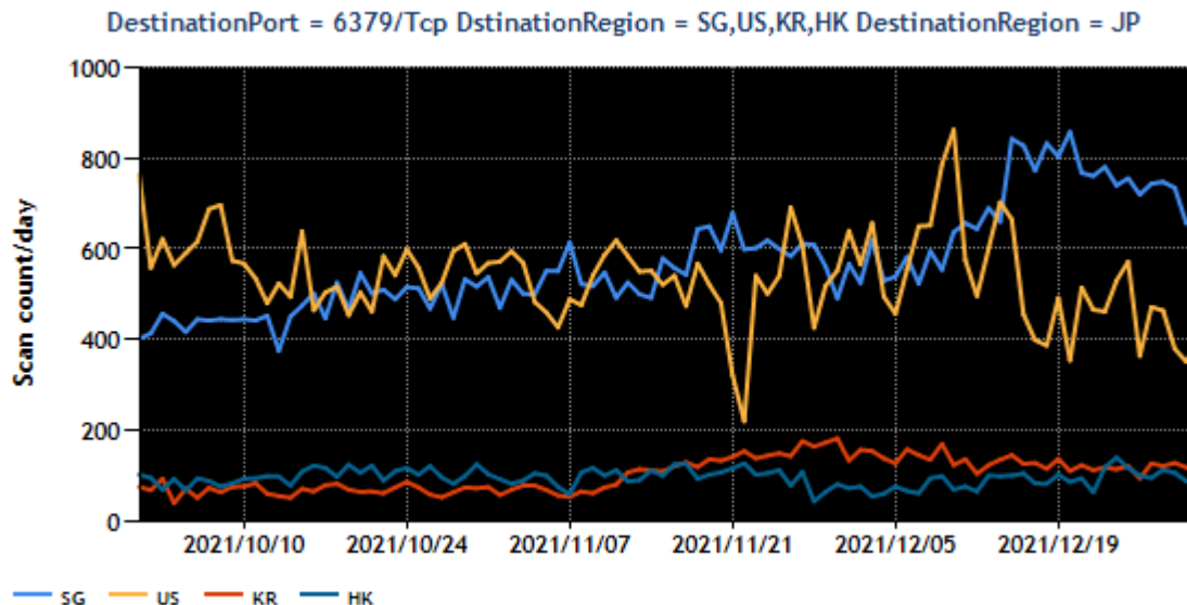
〔図 5：中国を除いた TOP2-5 を送信元地域とした Port6379/TCP 宛のパケット観測数の推移〕
